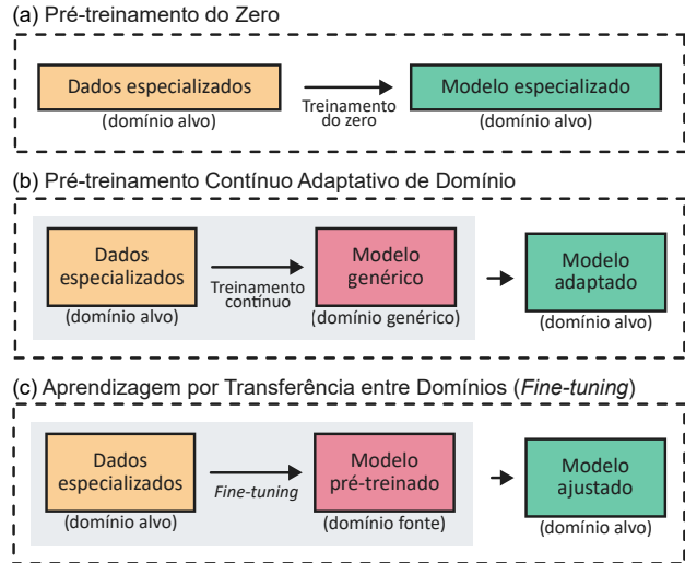
Figura 1: Estratégias de pré-treinamento.
