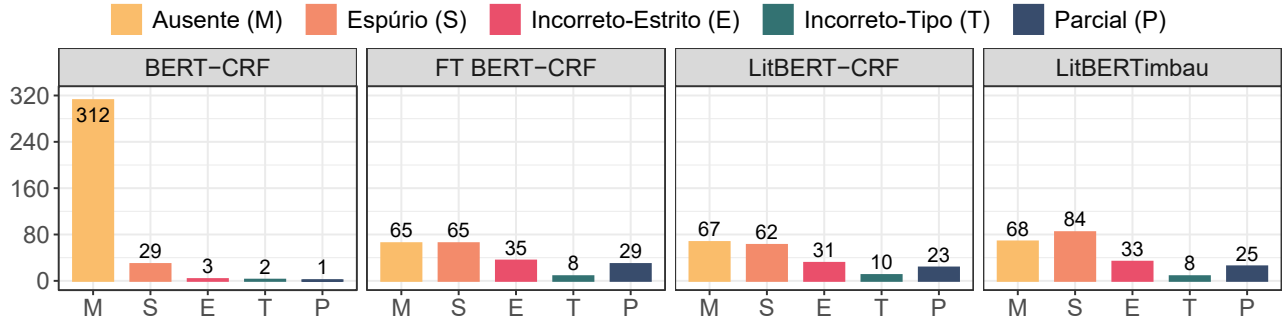
Figura 4: Distribuição de erros nos modelos avaliados.
