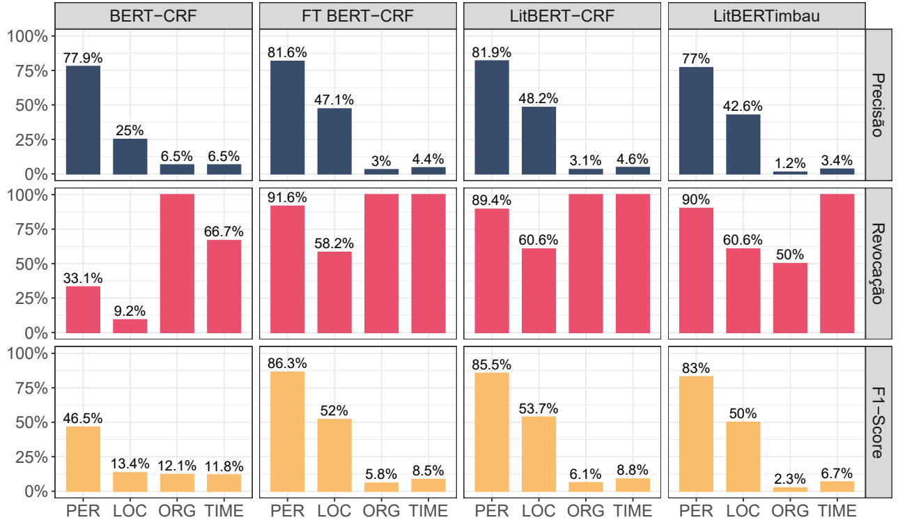
Figura 3: Métricas de avaliação para cada modelo, considerando o cenário tipo .
